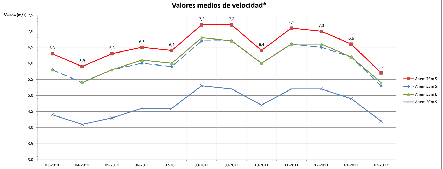
Velocidades medias* (m/s)
