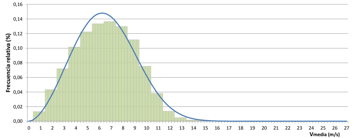
Distribución de frecuencia de Velocidad*
